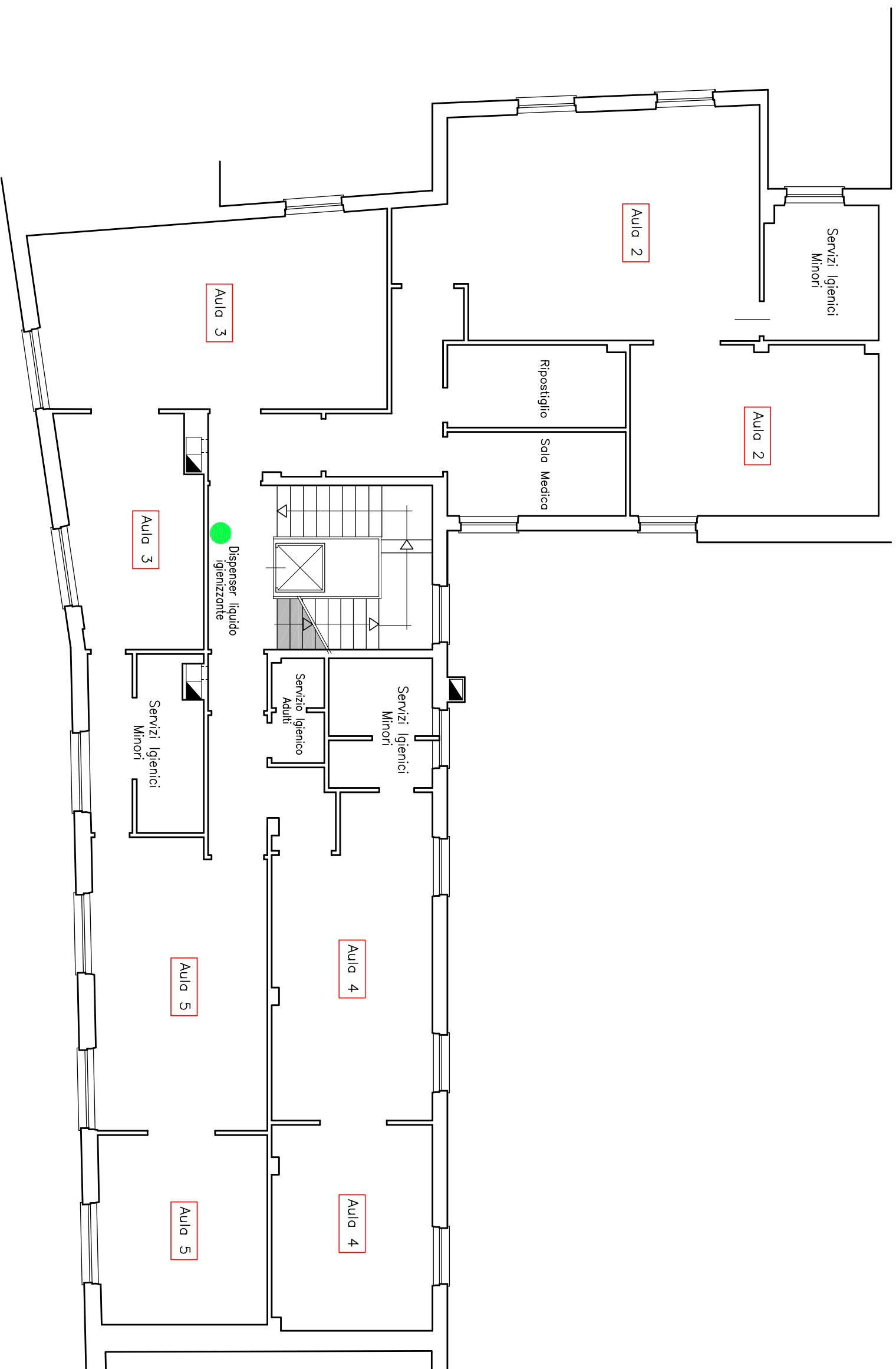
Pianta piano secondo Scala 1:100
